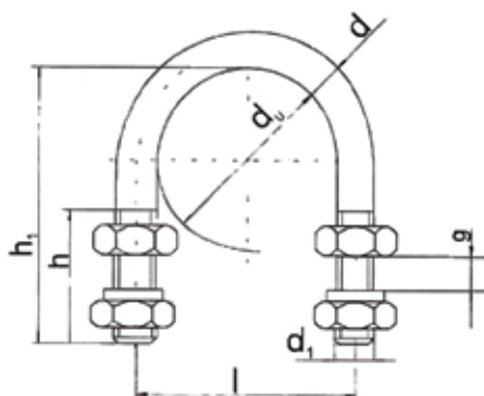
Obejmy do rur typ „E” (Rohrklemme)
